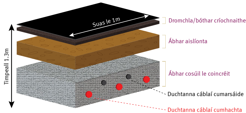
Fíor 5: Gnáthshocrú ducht le haghaidh cábla HVAC faoin talamh
