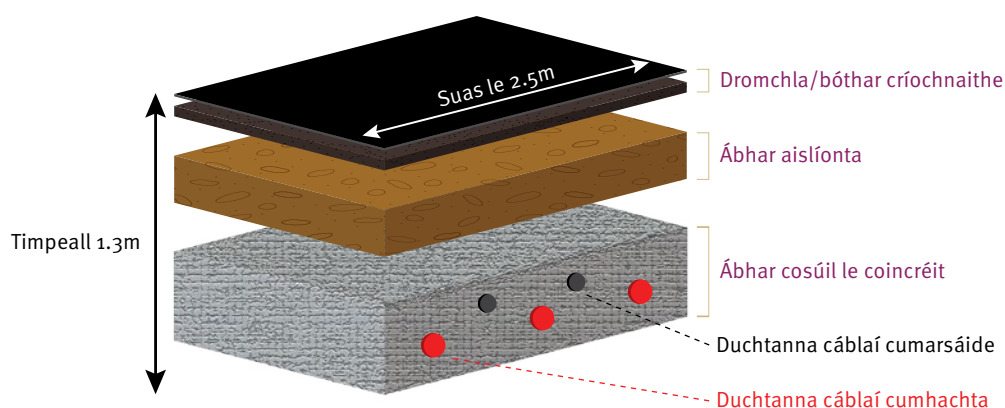
Fíor 9: Gnáthshocrú duchta le haghaidh cábla HVAC faoin talamh
