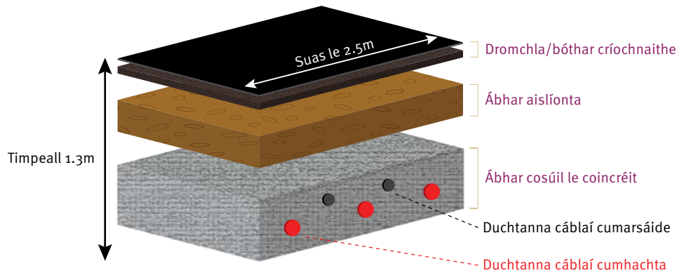
Fíor 4: Gnáthshocrú ducta le haghaidh cábla HVAC faoin talamh
