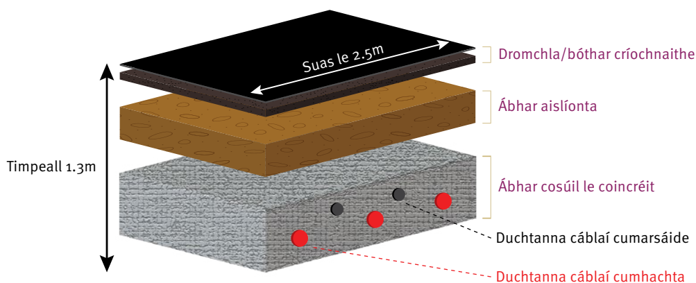
Fíor 3: Gnáthshocrú ducta le haghaidh cábla HVAC faoin talamh
