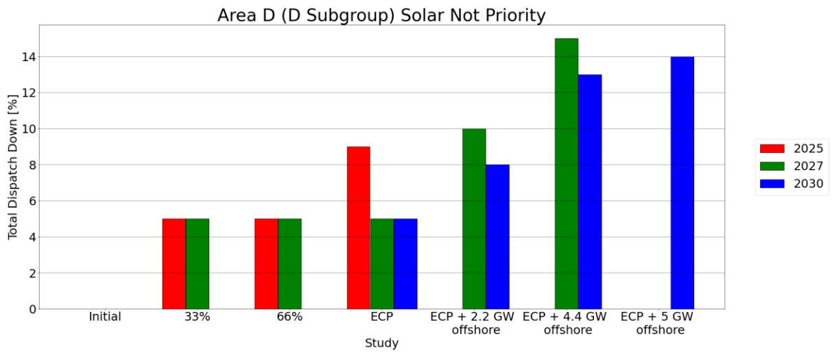
Figure 6-2 Results Solar Not Priority Area D (D)
