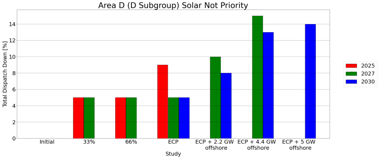
Figure 6-2 Results Solar Not Priority Area D (D)
