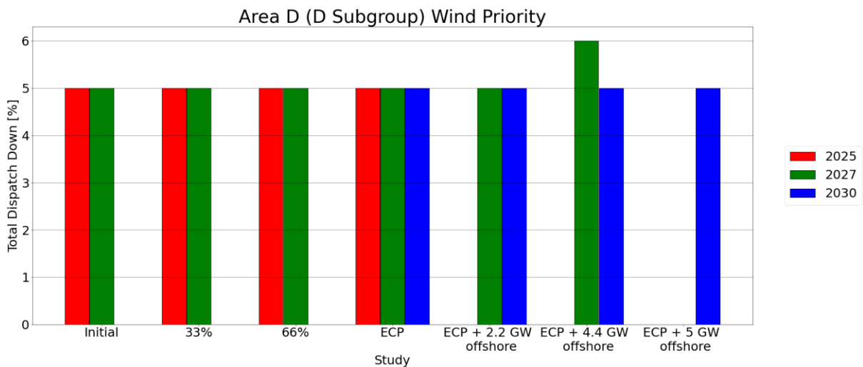
Figure 6-4 Results Wind Priority Area D (D)
