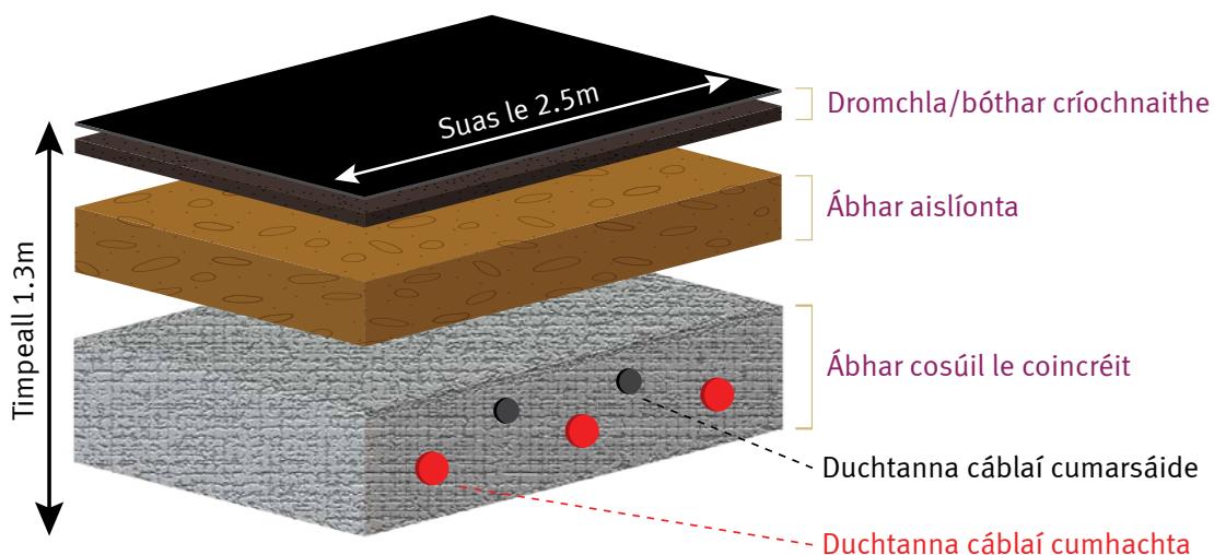
Fíor 4: Gnáthshocrú duchta cábla HVAC faoin talamh
